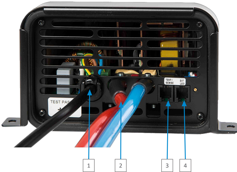
Abb. 3: ABC Anschlussseite mit Anschluss für die Sensorleitung CTS/TS und Fernanzeige
