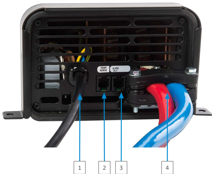
Abb. 2: ABC Anschlussseite mit Anschluss für CBL und Sensorleitung CTS/TS
