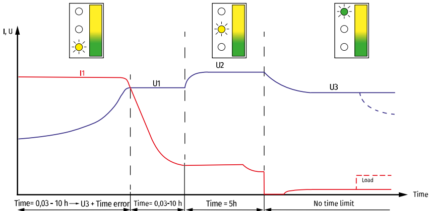
Abb. 4: Ladekennlinie Traktionsbatterie
