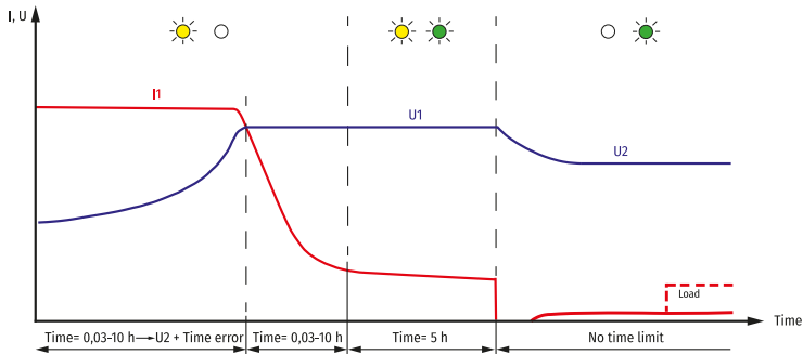
Abb. 2: IU1U2-Ladekennlinie
